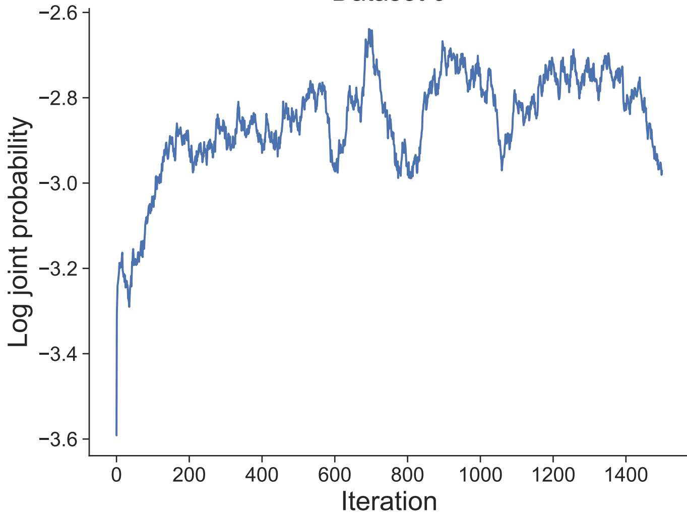
Dataset 0
