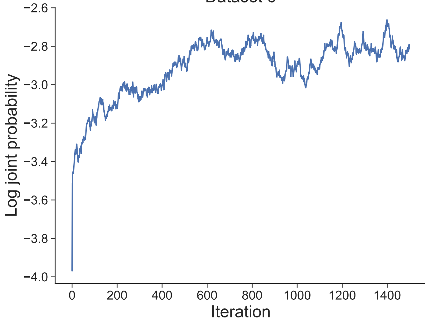
Dataset 6
