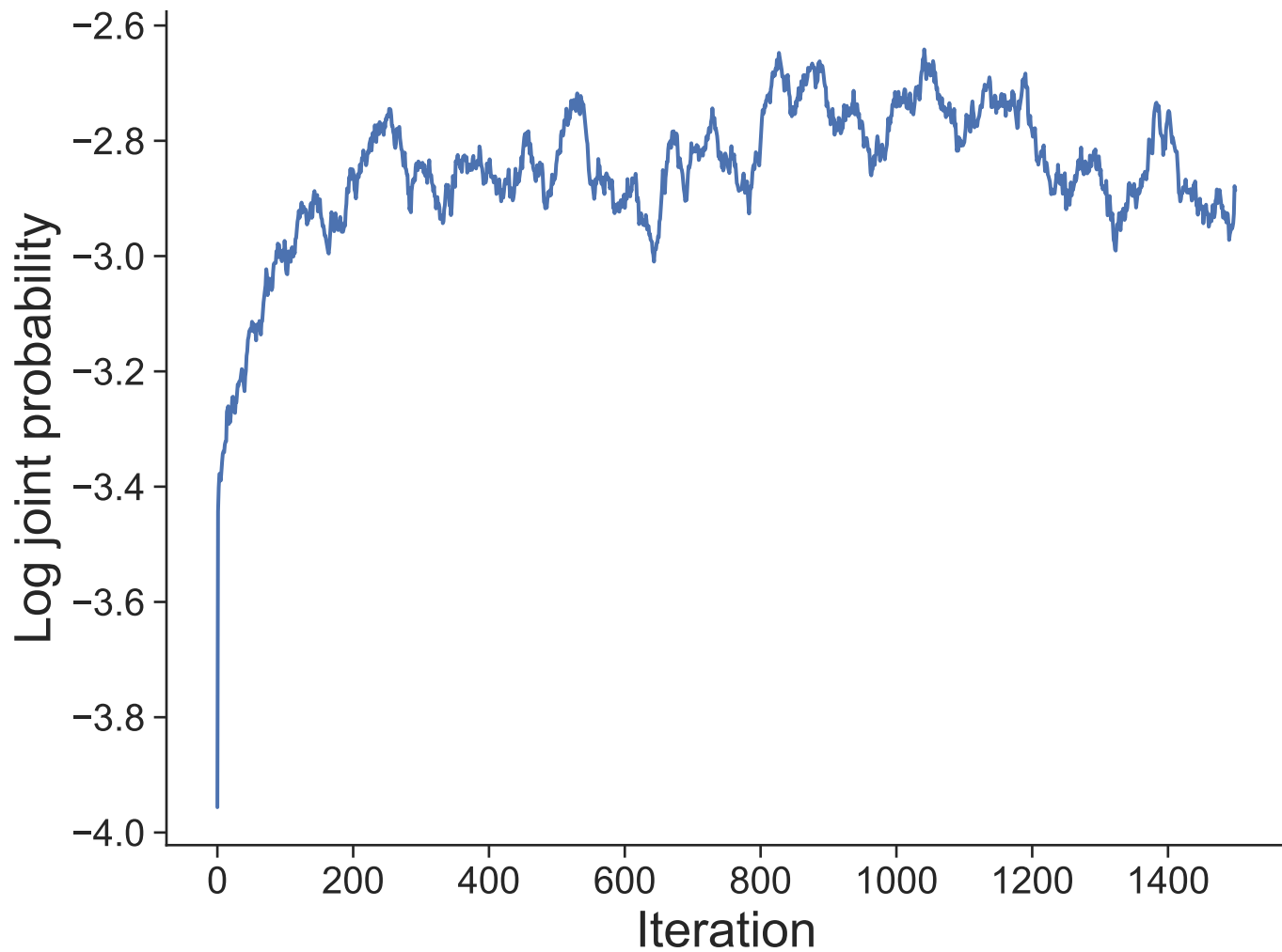
Dataset 47
